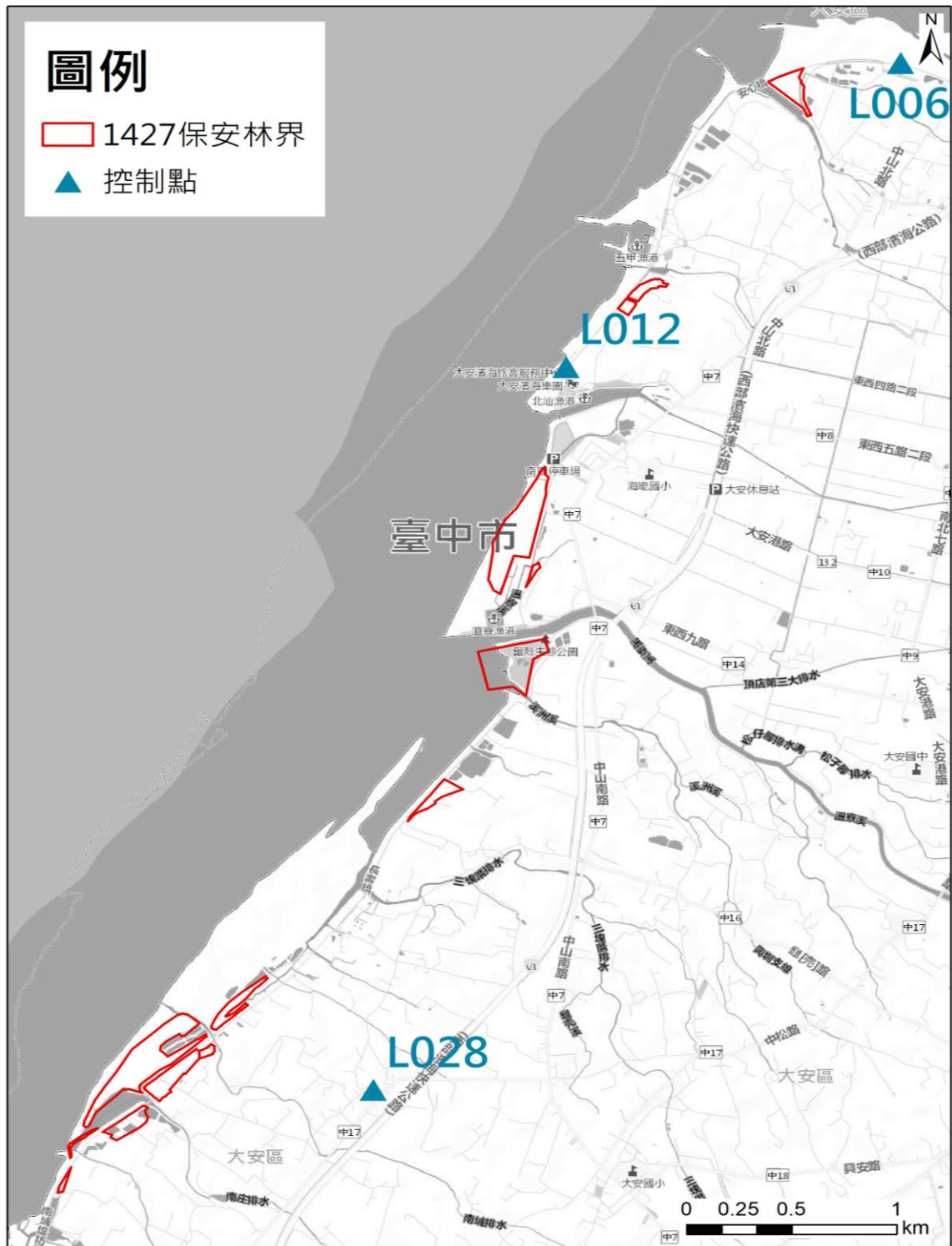
圖 12、GPS 控制點位置圖
