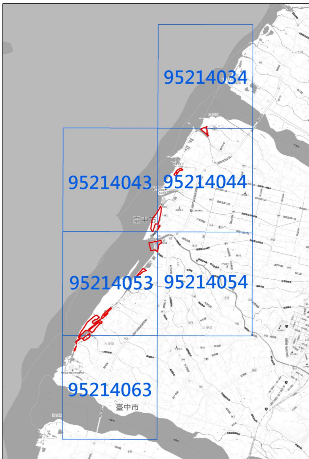
圖 11、保安林套疊正射影像圖幅接合圖
